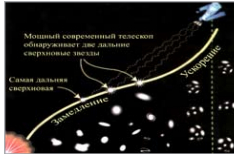
Рисунок, иллюстрирующий расширение Вселенной.
